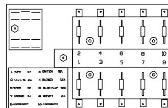
FUSES (FIG. 6.3.1)
